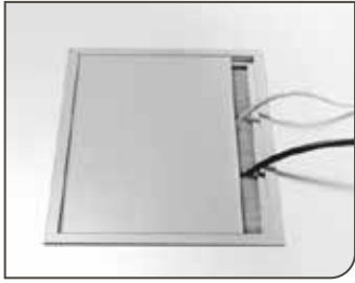
POWERBOX INBOUW. 24 x 12 CM. 3x RANDAARDE VOEDING, 2x DATA AANSL. WIT / ALU. EXCL. SNOER (BE011). BE001 213 €
